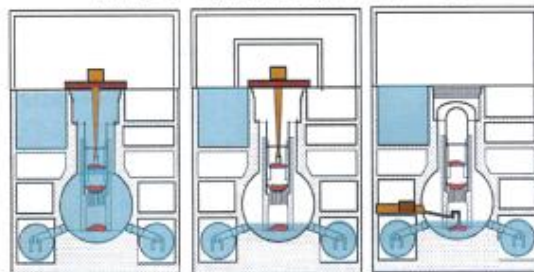
燃料デブリ取り出し工法(イメージ)
