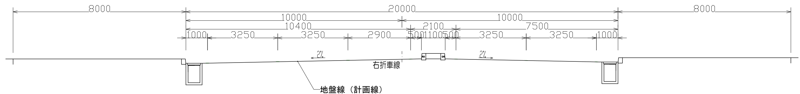
B 標準横断面図 (一般道路351号3・2・1長岡停車場線 (大手通り)) 幅員 W=20.0m
