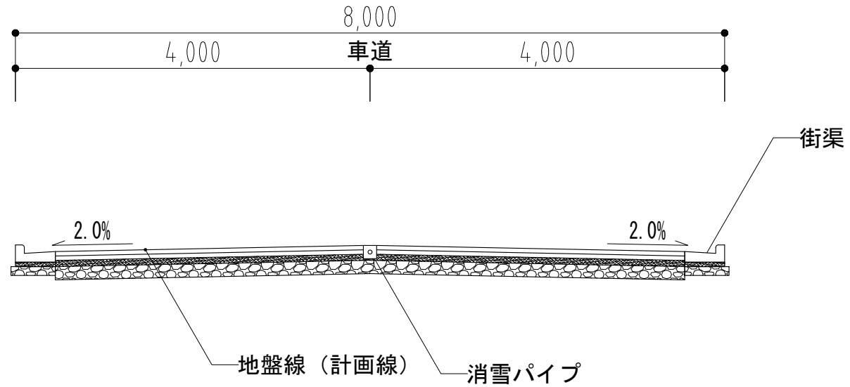
C標準横断面図 (市道406号線)
