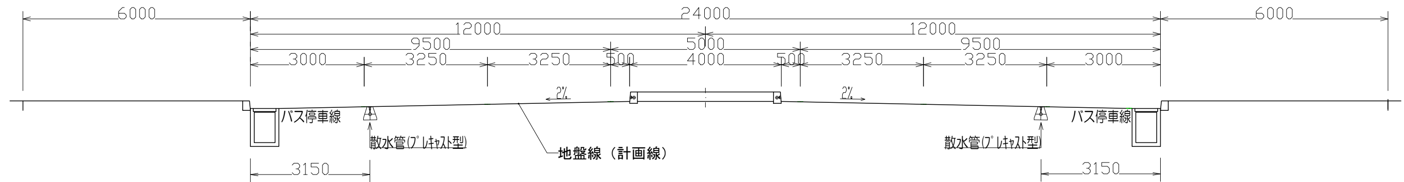
A 標準横断面図 (一般道路351号3・2・1長岡停車場線 (大手通り)) 幅員 W=24.0m
