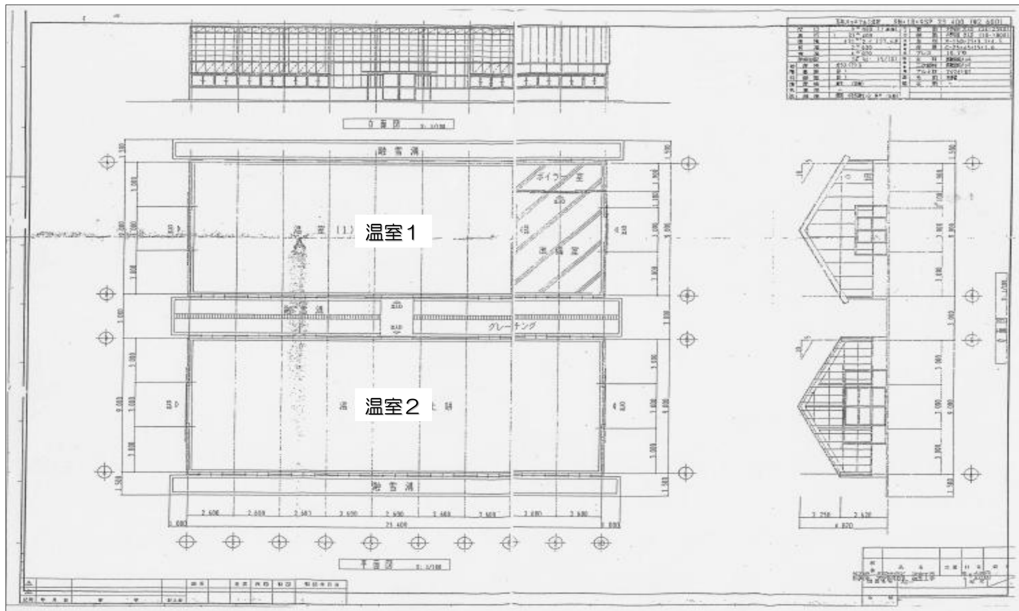
農業体験温室棟（温室1、温室2） 平面図
