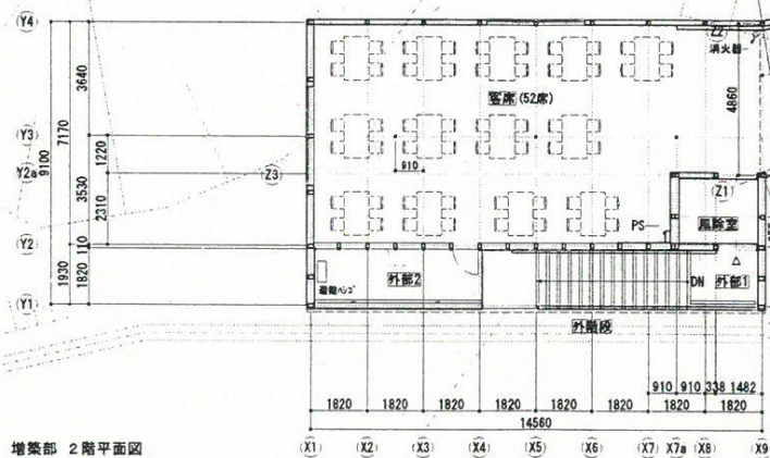
増築部 2階平面図
