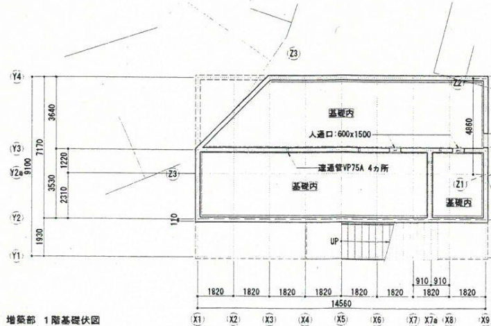
增築部 1階基礎伏図
