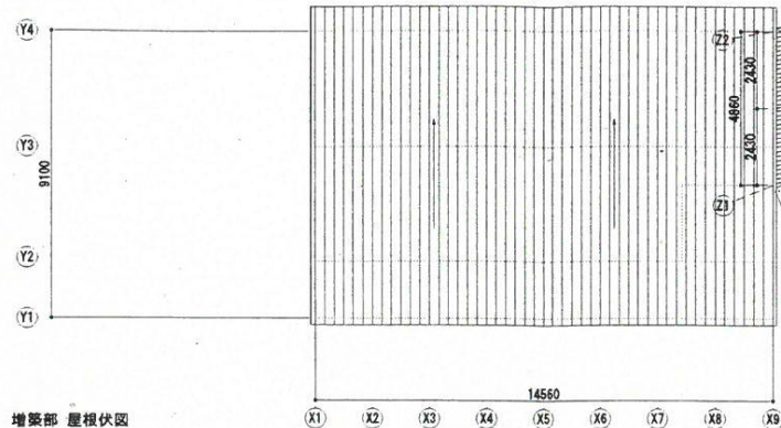
增築部 屋根伏図
