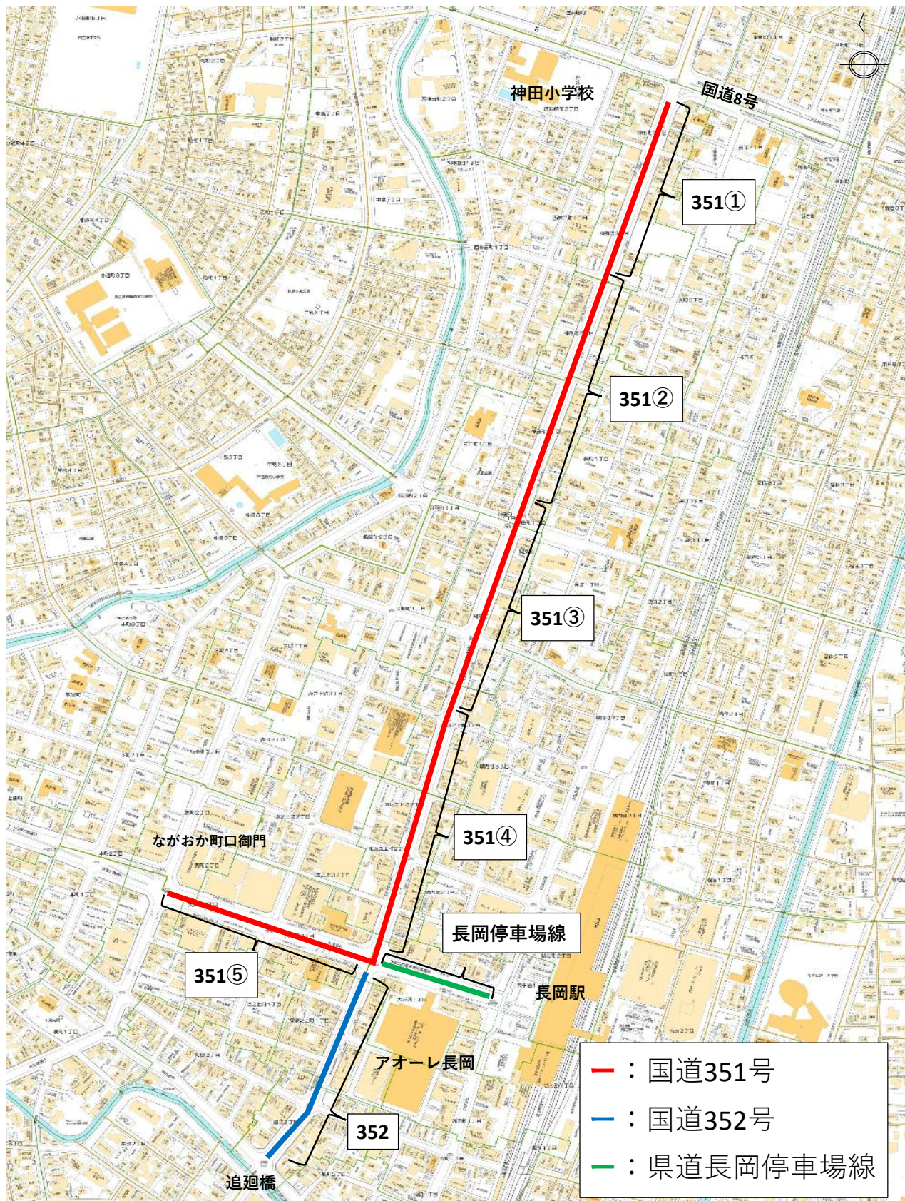
長岡市管理の国県道図面位置図（国道351号・国道352号・県道長岡停車場線）
