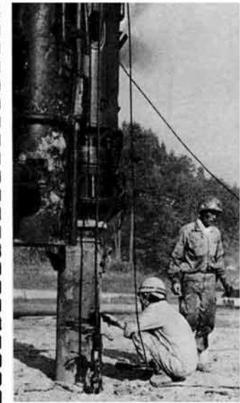
「くいうち」作業中の建設現場
