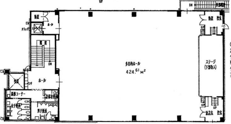
2階 平面図
